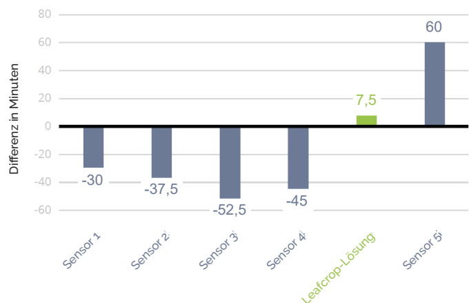
Zeitdifferenz zwischen der realen und gemessenen Dauer der Blattnässe
