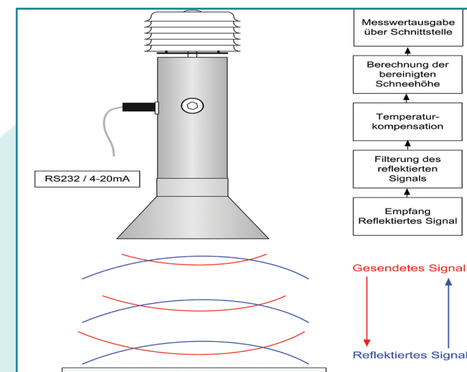
Abb. 1: Signalverarbeitung des USH-8 Schneehöhensensors.
